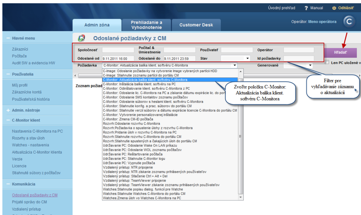
Obrázok č. 7 Vojdite do Požiadaviek a zvolte „Odoslanie aktualizáčného balíka klient. softvéru C-Monitora. Vypĺňte filter podľa vašich kritérií.
