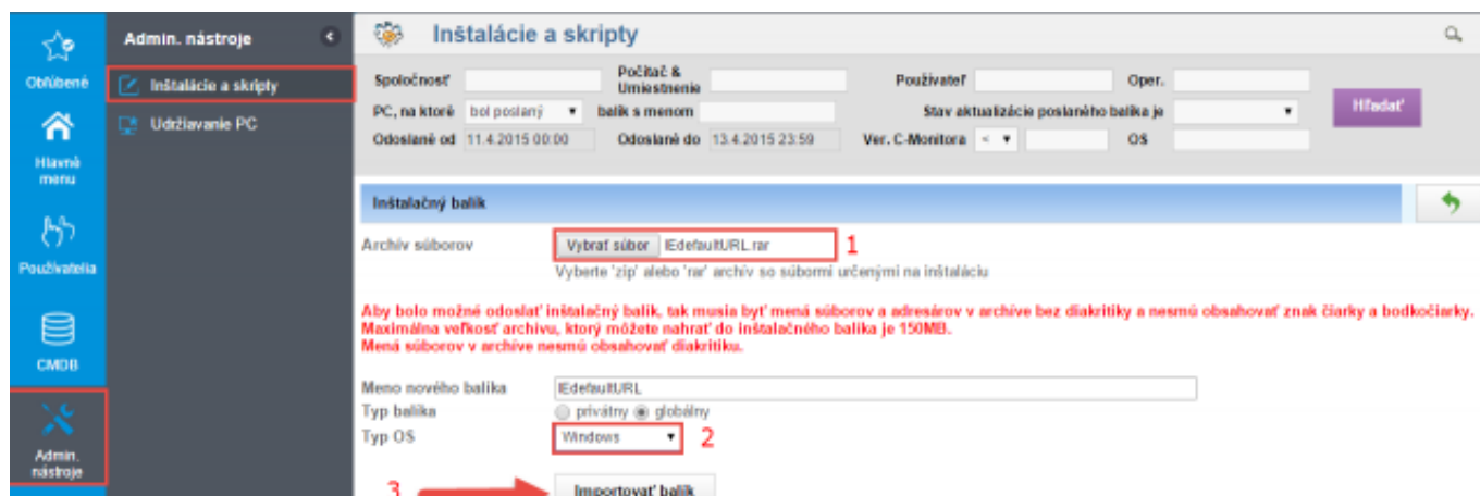
Obrázok: Import balíka pre distribúciu do C-Monitor klientov
