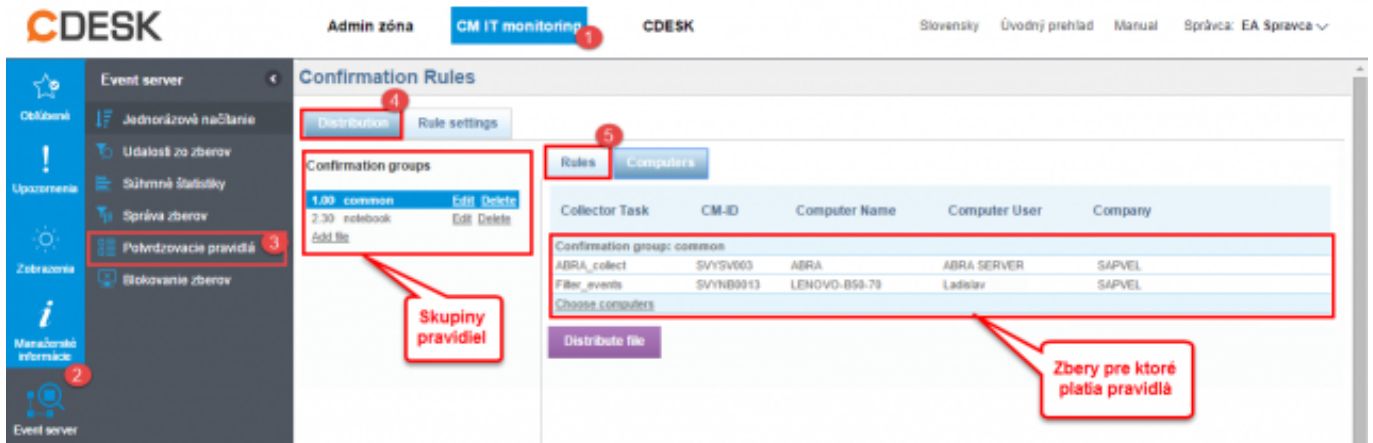
Obrázok: Zobrazenie a konfigurácia počítačov patriacich k pravidlu
